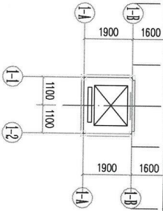
底层电梯平面布置图
