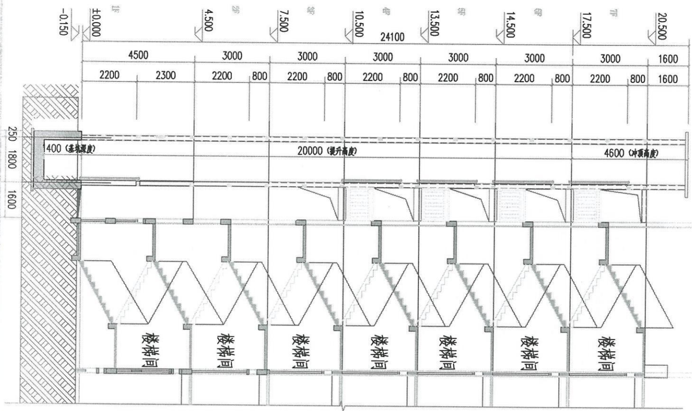
剖面图 1:100
